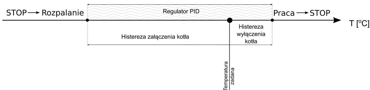
Ilustracja 20: Schemat przełączania się algorytmu spalania między mocami dla regulatora procesu spalania PID
