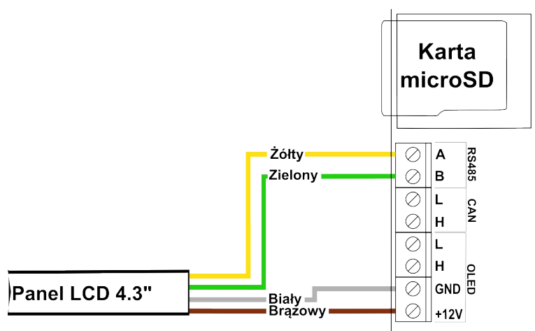
Ilustracja 2: Podłączenie panelu CDI 4.3" w sterowniku Pello
