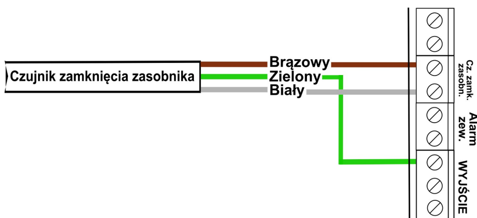
Ilustracja 6: Podłączenie czujnika zamknięcia zasobnika
