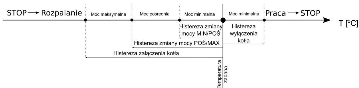
Ilustracja 19: Schemat przełączania się algorytmu spalania między mocami dla regulatora procesu spalania Auto
