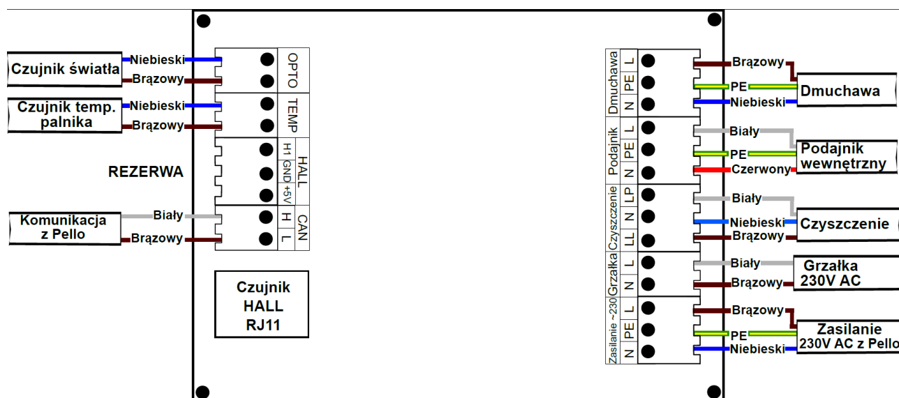
Ilustracja 3: Podłączenie na płytce elektronicznej w palniku
