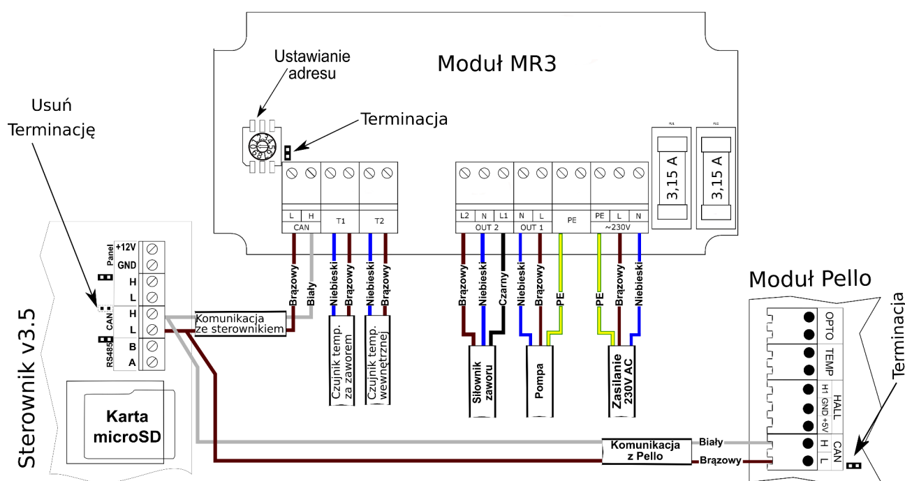
Ilustracja 8: Schemat podłączenia modułu rozszerzeń MR3.
